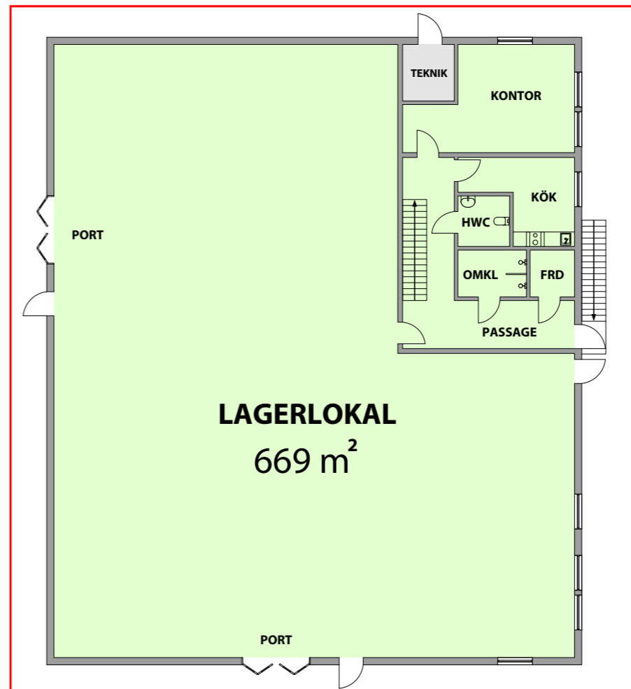
ENTRÉPLAN
