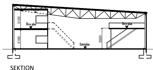
SEKTION
